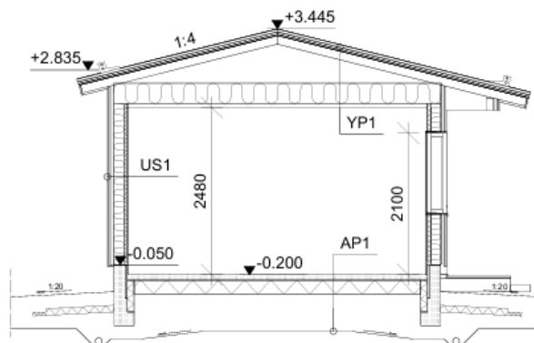
LEIKKAUS A-A
